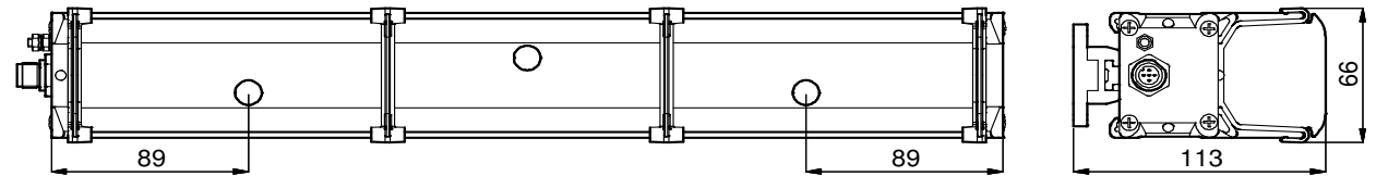
Zeichnung ThunderION 2.0
